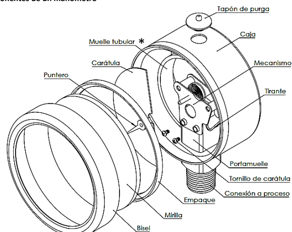
Componentes de un manómetro
