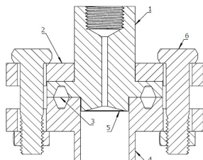
Simulación de montaje sello químico serie 220 con brida RTJ
