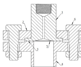
Simulación de montaje sello químico serie 220 con brida RF
